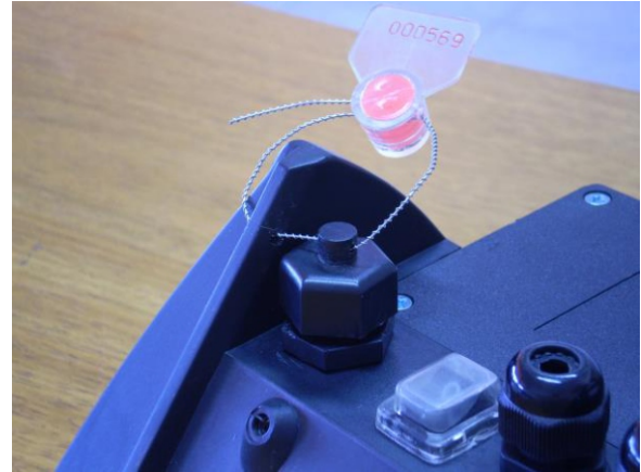
FIGURA 14. Acceso al pulsador de calibración en el gabinete inoxidable
